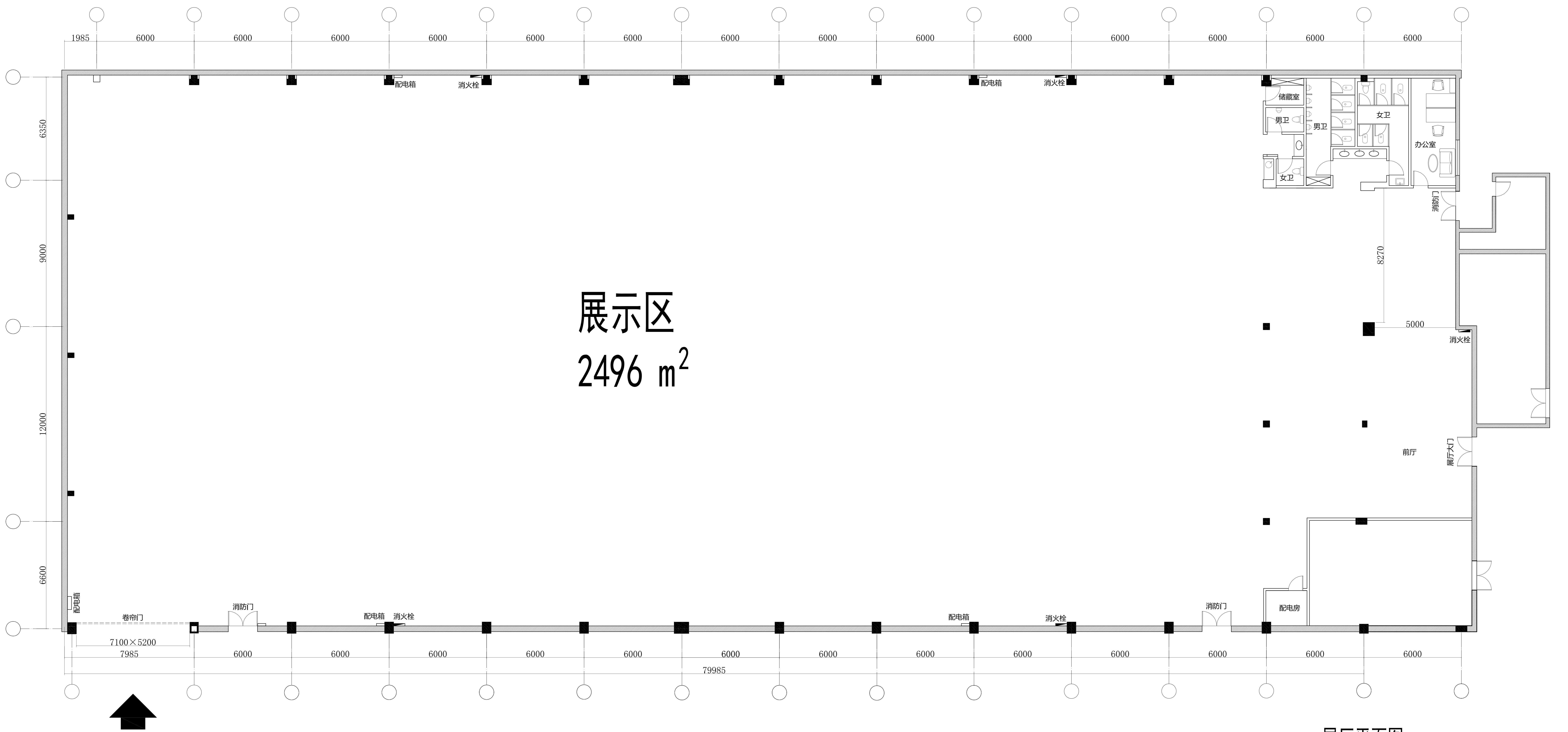
展厅平面图 1:100
